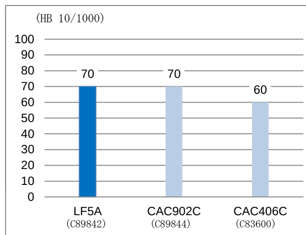
图 8 布氏硬度
