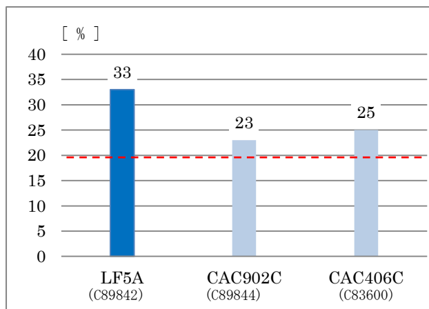
图 7 伸长率
